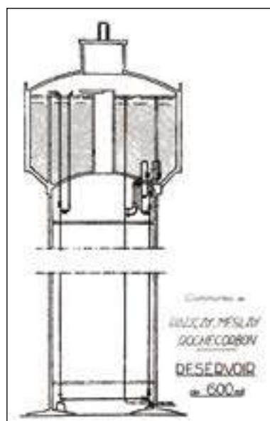
Plan schématique du château d'eau : c'est un réservoir de 600 000 litres d'eau. L'ensemble est d'une hauteur totale de 44 mètres. Sa fonction est de réguler la pression et le débit de l'eau.
